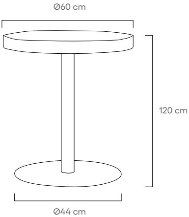
Tavolo Mattei tondo realizzato in multistrato 4 cm con bordo e piano in ABS+SAN Balance® Versalis e struttura in acciaio satinato. Dimensioni: ø60 cm / h120 cm / Base ø44 cm
